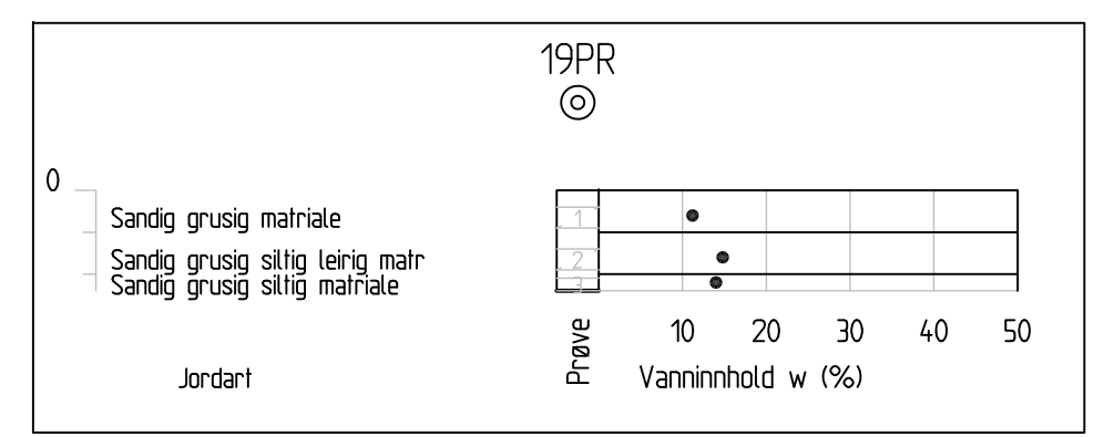
Profil 150 1 : 200
