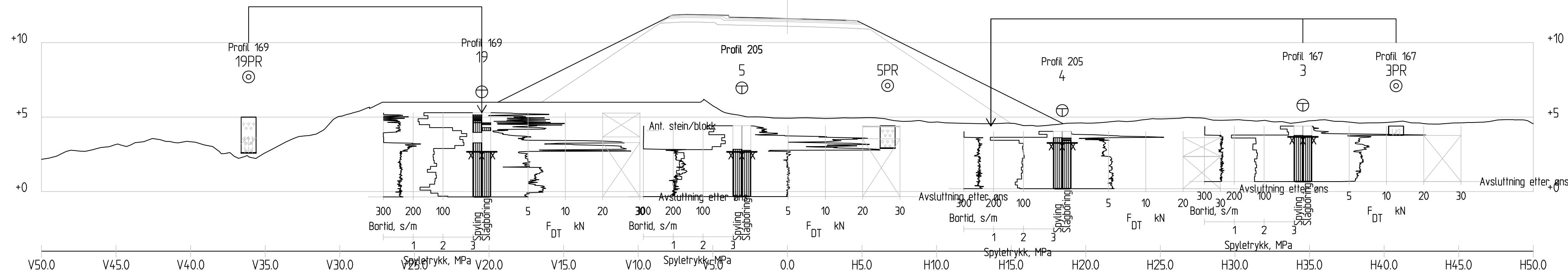
Profil 200 1 : 200
